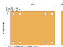
Dimension des blocs de renforts bois
