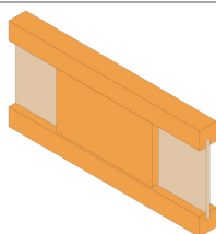
Installation d'un renfort bois sur un support poutre en I
