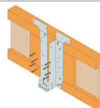
Fixation par les brides latérales sur un support poutre en I avec renfort
