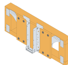
Fixation par les brides supérieures sur une poutre métallique ajourée avec renfort bois
