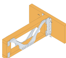
Fixation d'une poutre métallique ajourée par les brides latérales sur un support bois massif
