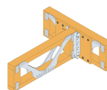
Fixation par les brides latérales sur une poutre métallique ajourée avec renfort bois
