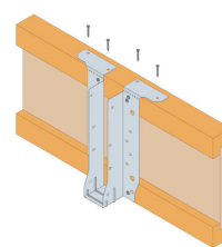
Fixation par les brides supérieures sur un support poutre en I
